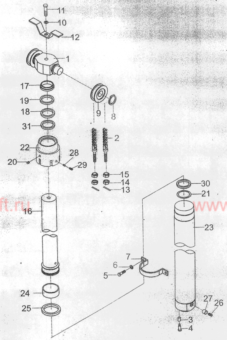
图64/FIG. 64 前起升油缸 (二级全自由 3.5t) /FRONT LIFT CYLINDER (FULL FREE 2-STAGE MAST ZM)
