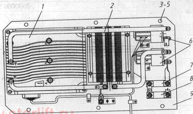
图 51 控制器 (AC) CPD10-35J C1 Fig. 51 Controller (AC) CPD10-35J C1
