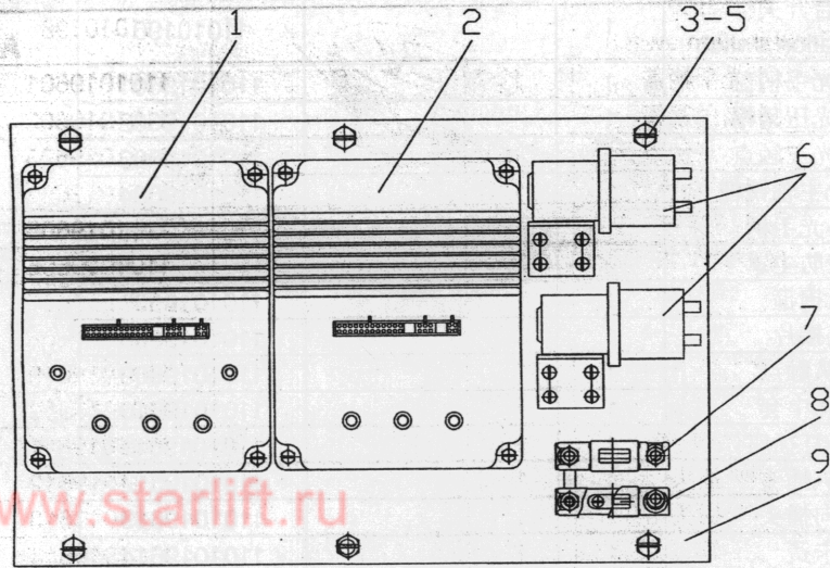
图 49 控制器 (DC) CPD10-30J Fig. 49 Controller (DC) CPD10-30J
